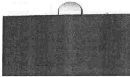
Gambar 3. Sudut kontak specimen S8A2 pada penyinaran UV 24 jam
