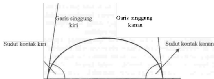
Gambar 1. Pengujian sudut kontak: hidrofobik
