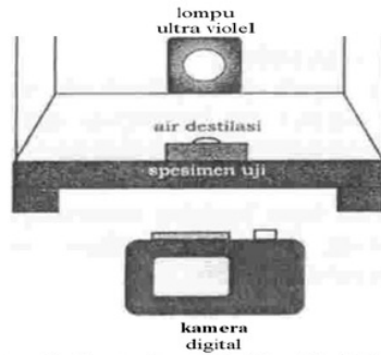
Gambar 1. Pengujian sudut kontak: hidrofobik
